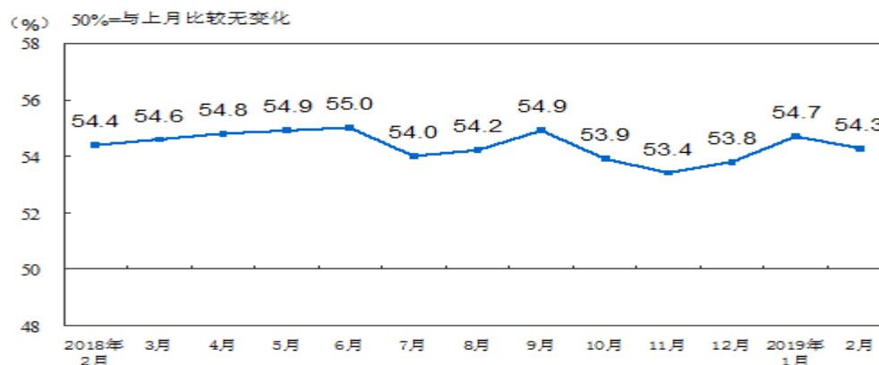
图2 非制造业商务活动指数（经季节调整）
